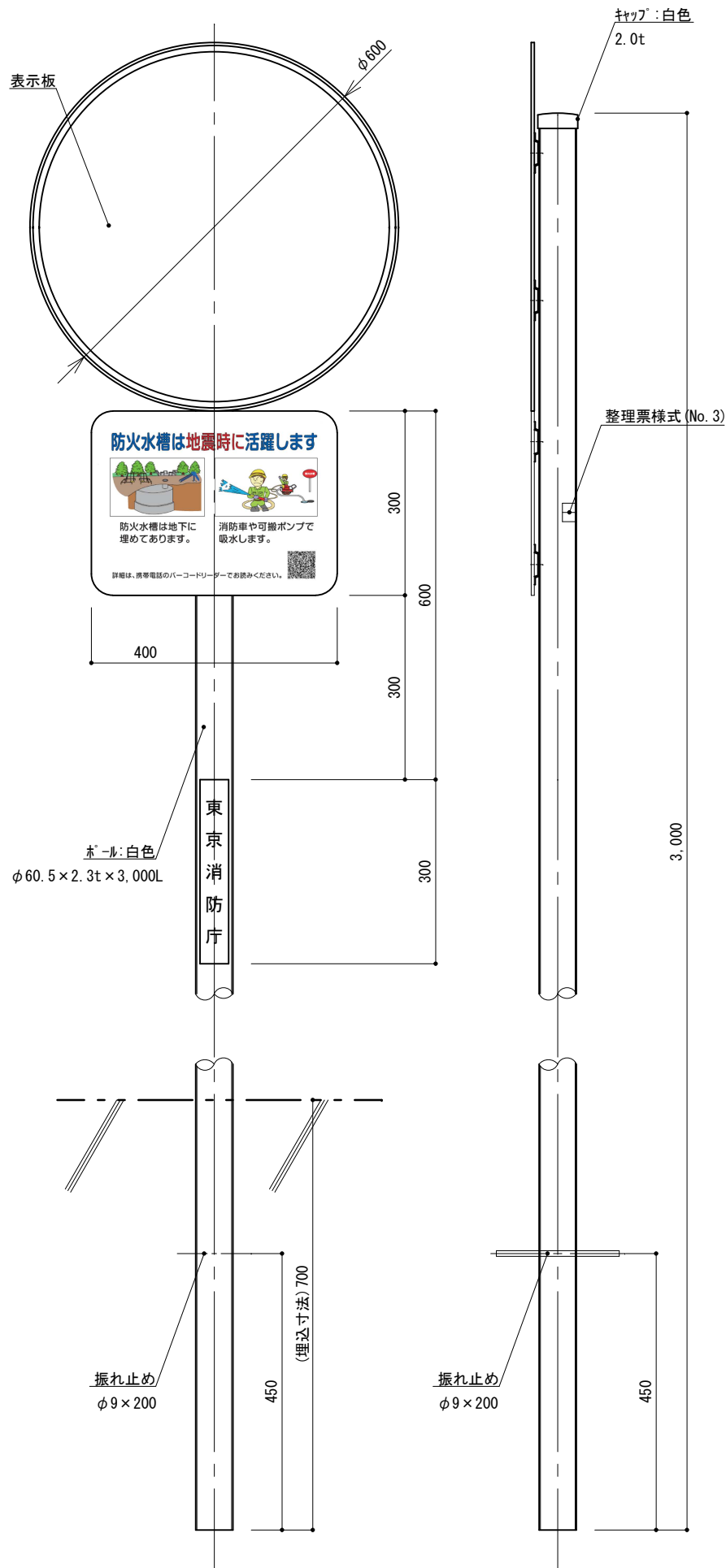
ホ-ル部詳細図
