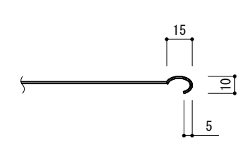
外縁処理
