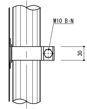
取付金具
