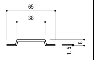
補強リブ
