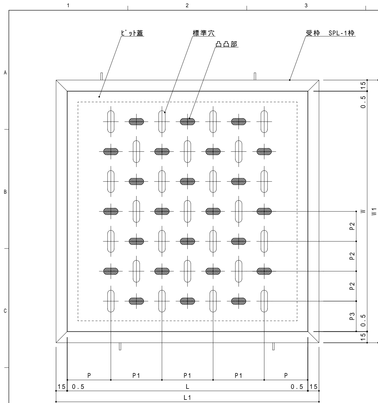
【標準寸法】
