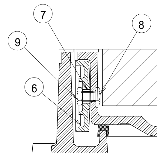
断面Z-Z
