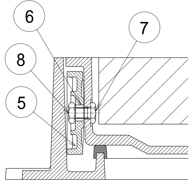
断面Z-Z
